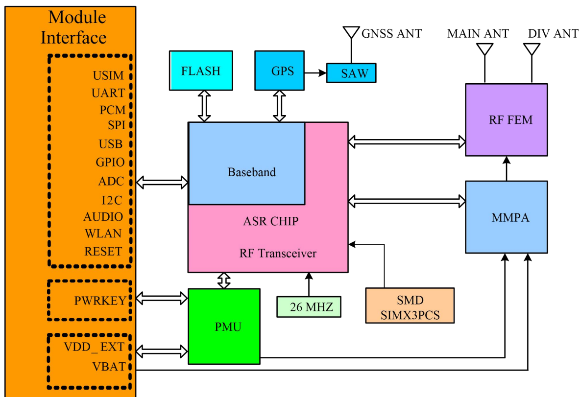
图2-1 CLM920_JC3 LCC模块功能框图
