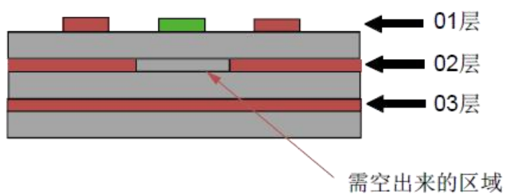
图 3-36 参考地为第三层 PCB 微带传输线结构
