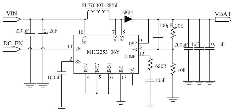
图 3-4 DC/DC 开关电源参考电路
