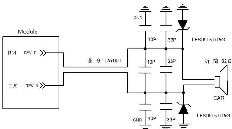
图3-30 音频输出参考电路
