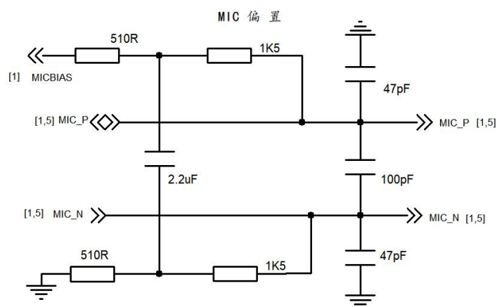
图 3-29 麦克风偏置电压参考电路
