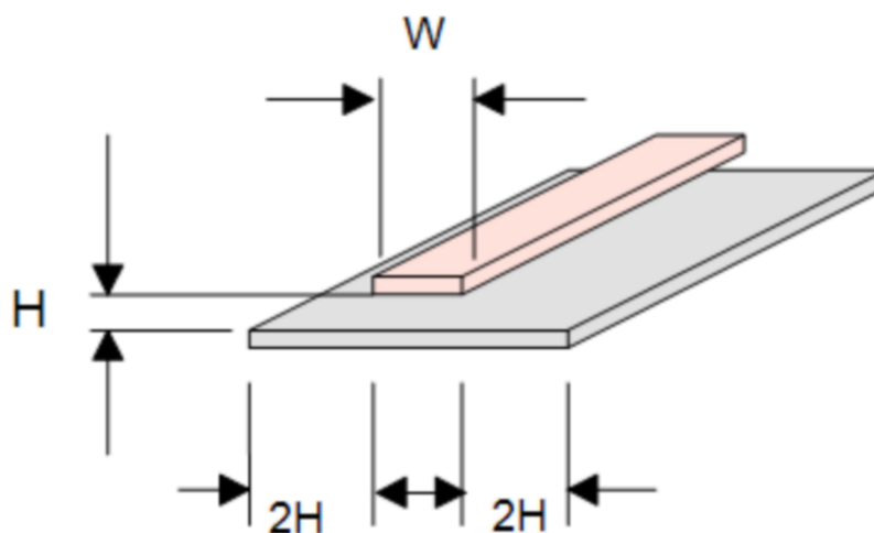
图 3-34 微带线的完整结构
