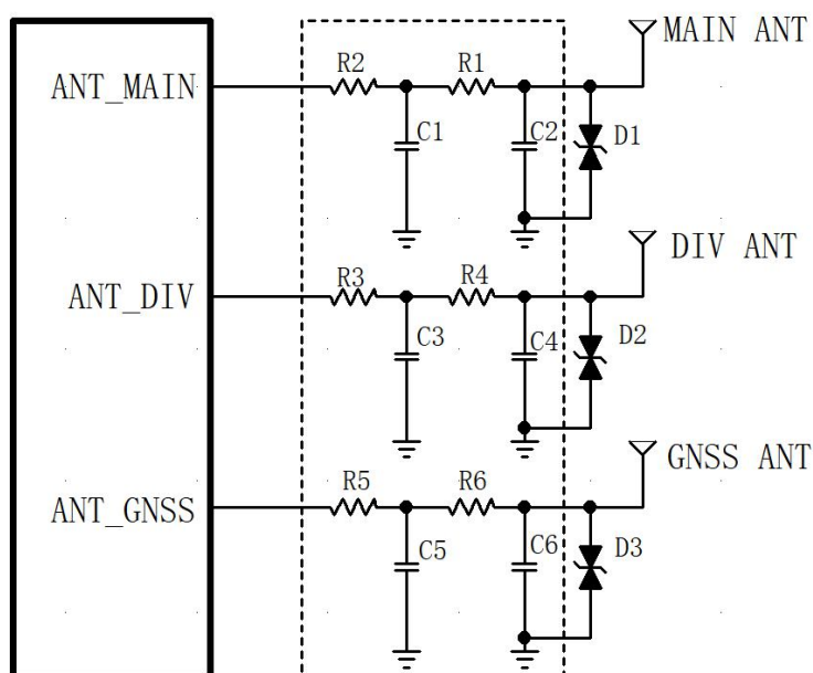
图 3-32 天线匹配电路
