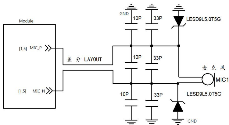
图 3-28 麦克风语音输入参考电路
