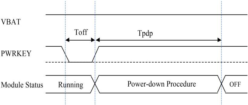
图 3-9 关机时序图
