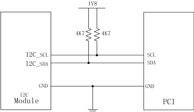
图 3-26 I2C 接口参考电路图
