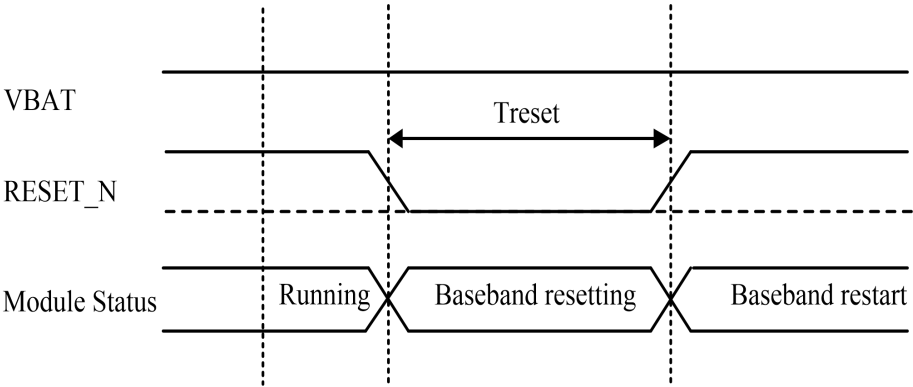
图 3-12 复位时序图
