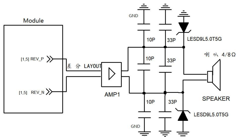
图 3-31 音频放大输出参考电路
