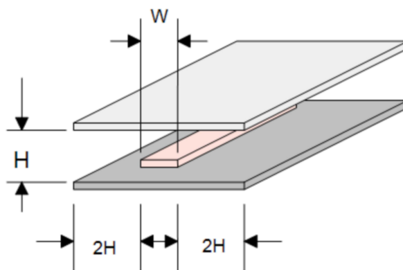
图 3-35 带状线的完整结构
