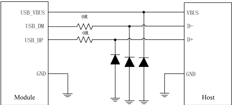
图 3-17 USB 连接设计电路图
