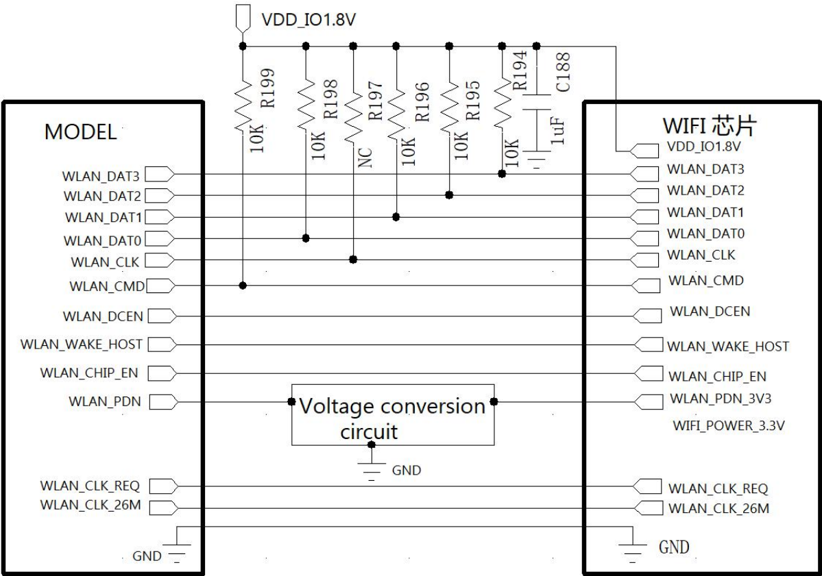
图 3-27 WLAN 接口参考电路图
