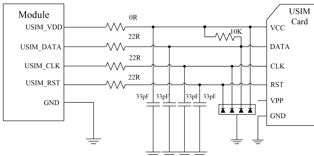
图3-21 USIM设计电路图
