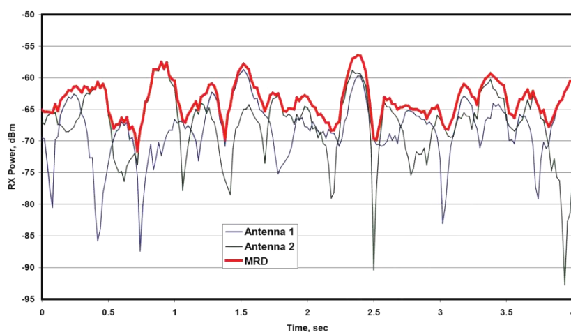
图 3-33 带分集和不带分集天线接收信号强度比较
