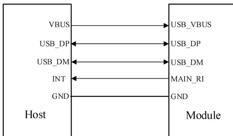
图 3-15C 支持 MAIN_RI 唤醒功能硬件连接图
