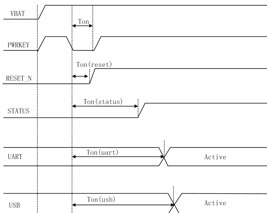
图 3-8 开机时序图
