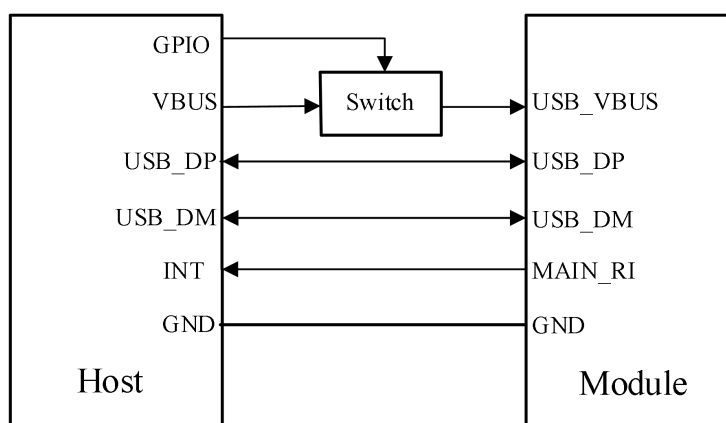
图 3-15D 不支持 USB 挂起功能硬件连接图上
