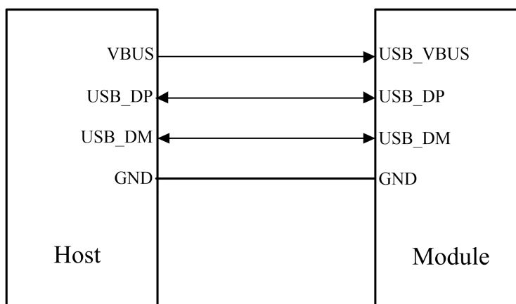
图 3-15B 支持 USB 远程唤醒功能硬件连接图
