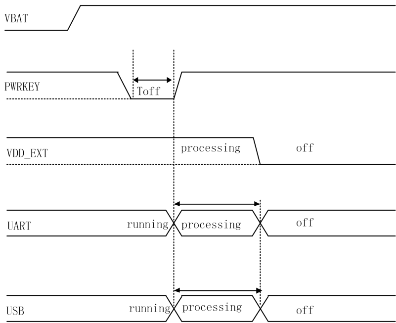
图 3-11 关机时序图
