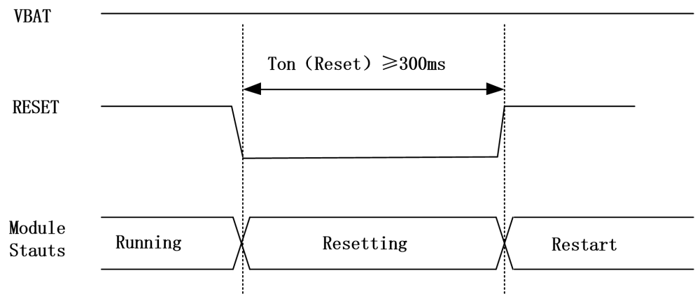
图 3-7 复位时序图
