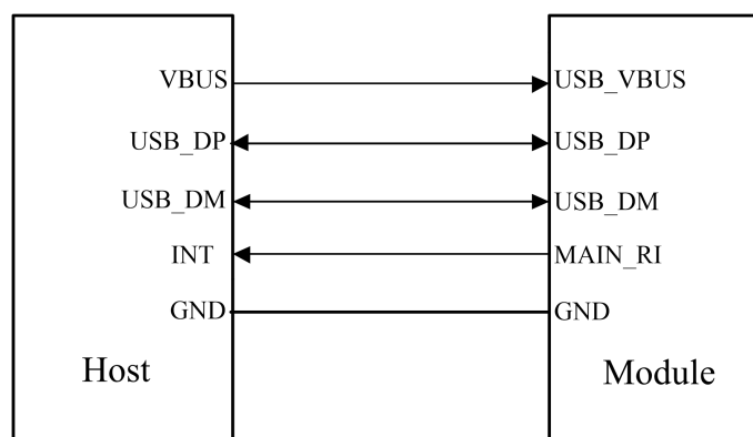
图 3-15C 支持 MAIN_RI 唤醒功能硬件连接图
